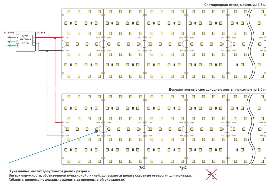
Схема 1. Подключение нескольких светодиодных лент
