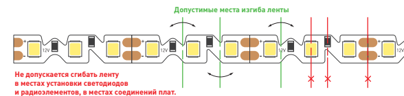
Рис. 5. Места сгиба ленты
